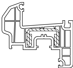
Армирование 35 x 20
