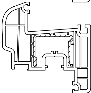
Армирование 35 x 28
