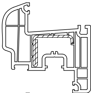
Армирование 35,5 x 28
